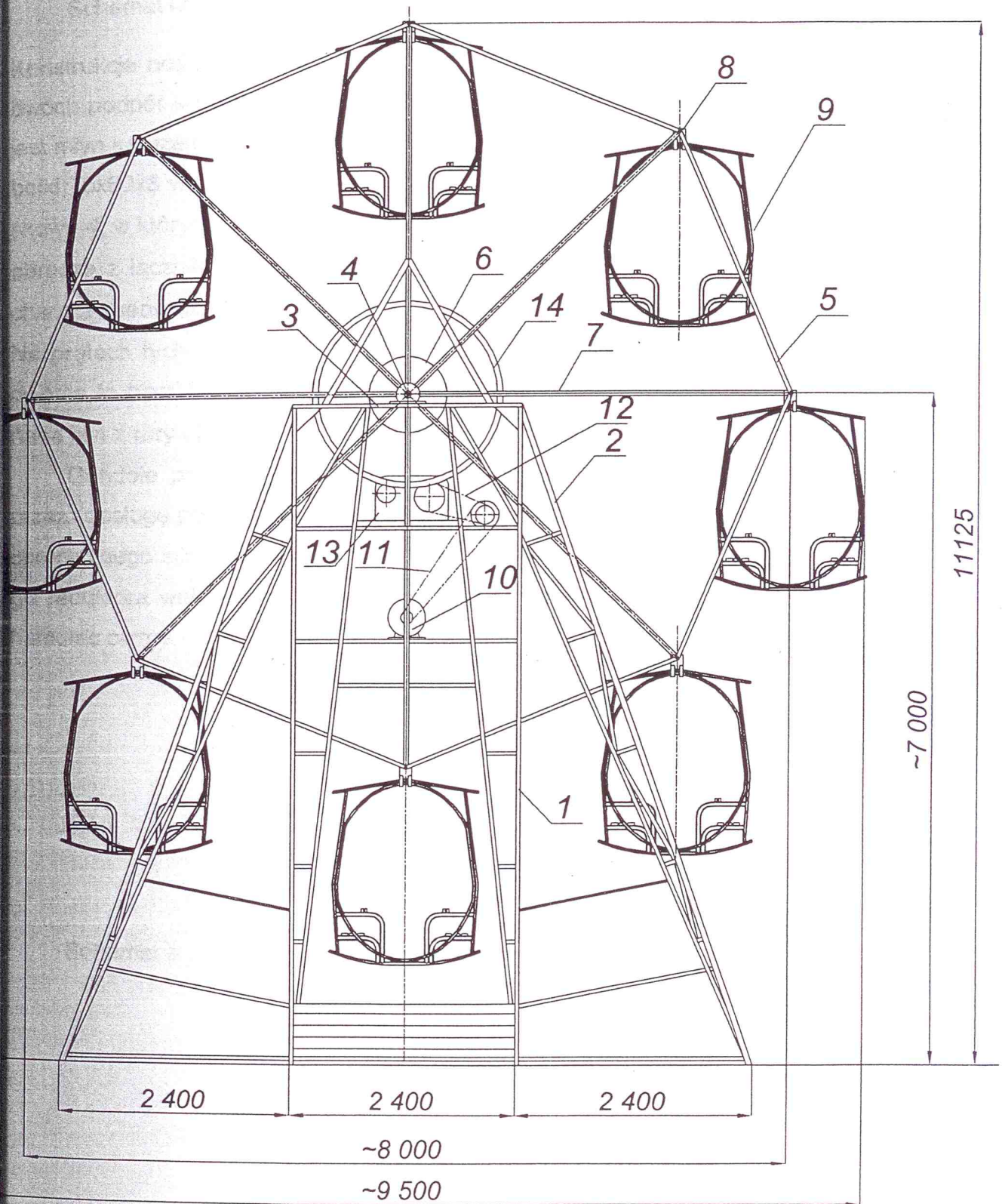
Rys 1. Schemat konstrukcji karuzeli
