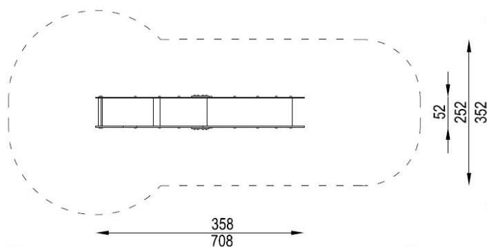
Rzut urządzenia wraz ze strefą funkcjonalną
